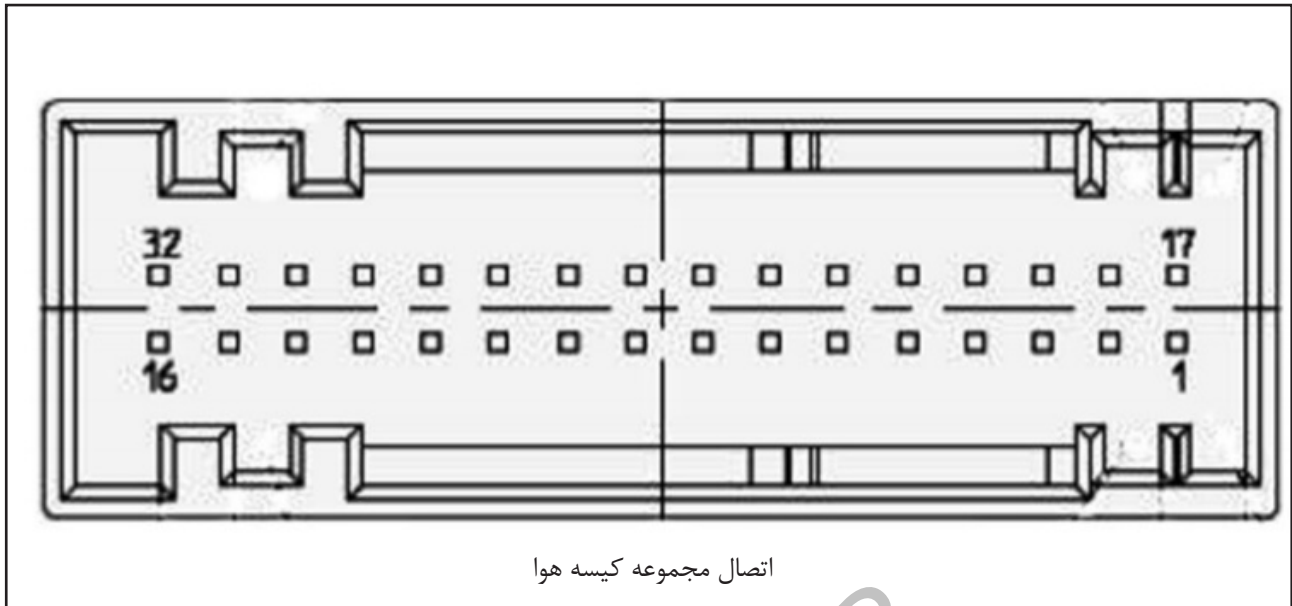
نقشه پین‌های اتصال مجموعه کیسه هوا
